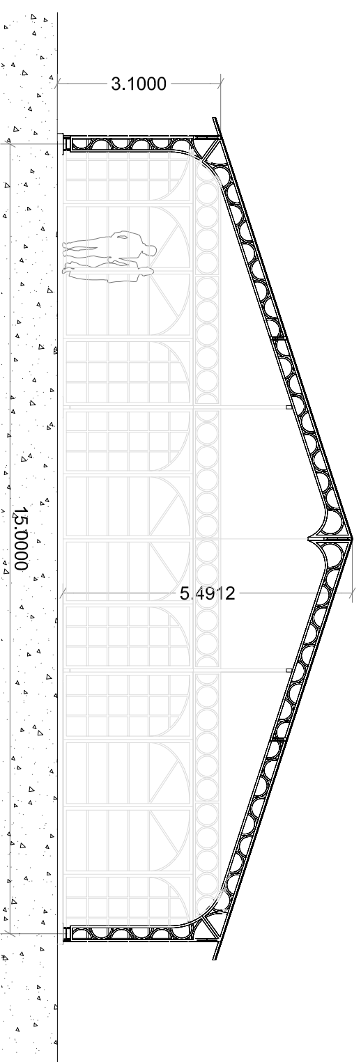
SEZIONE A-A
