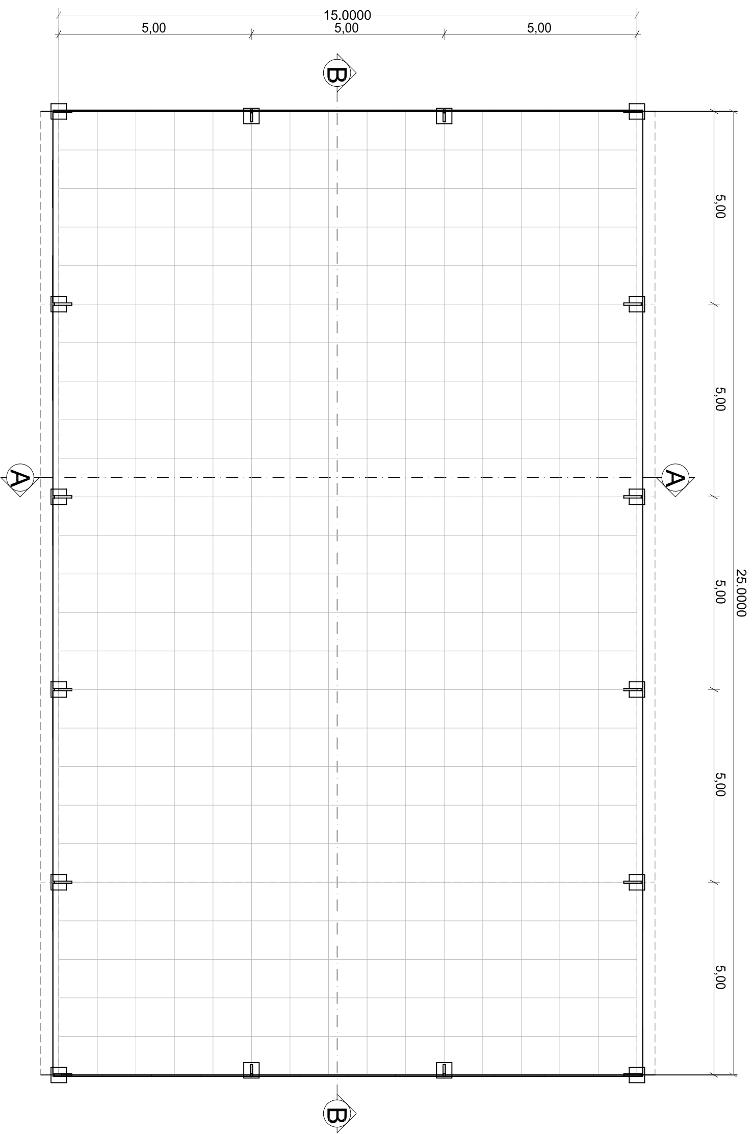
Pianta Padiglione
